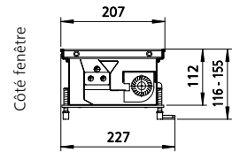
Vue transversale (exemple avec grille à enrouler)
